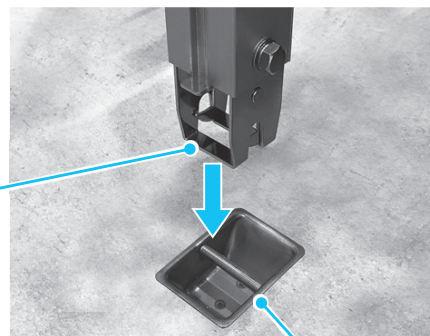
アンカー
