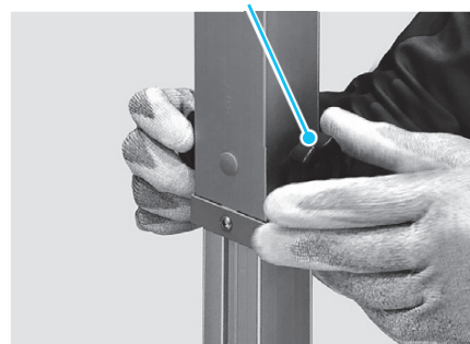
ノブナット
