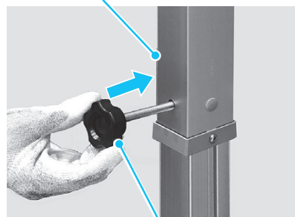
ノブボルト
